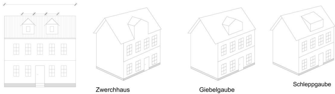
Abb. 1: Die Breite der Dachaufbauten darf max. 2/3 der Fassadenbreite betragen. Dachaufbauten müssen mind. 1 m Abstand untereinander und zur Gebäudeaußenkante halten.
